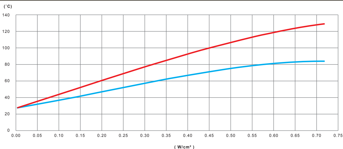
Variation, en fonction de la puissance en W/cm² du ruban chauffant en silicone, de la température de paroi d'un tube en PVC rempli d'eau non circulante, non isolé thermiquement
