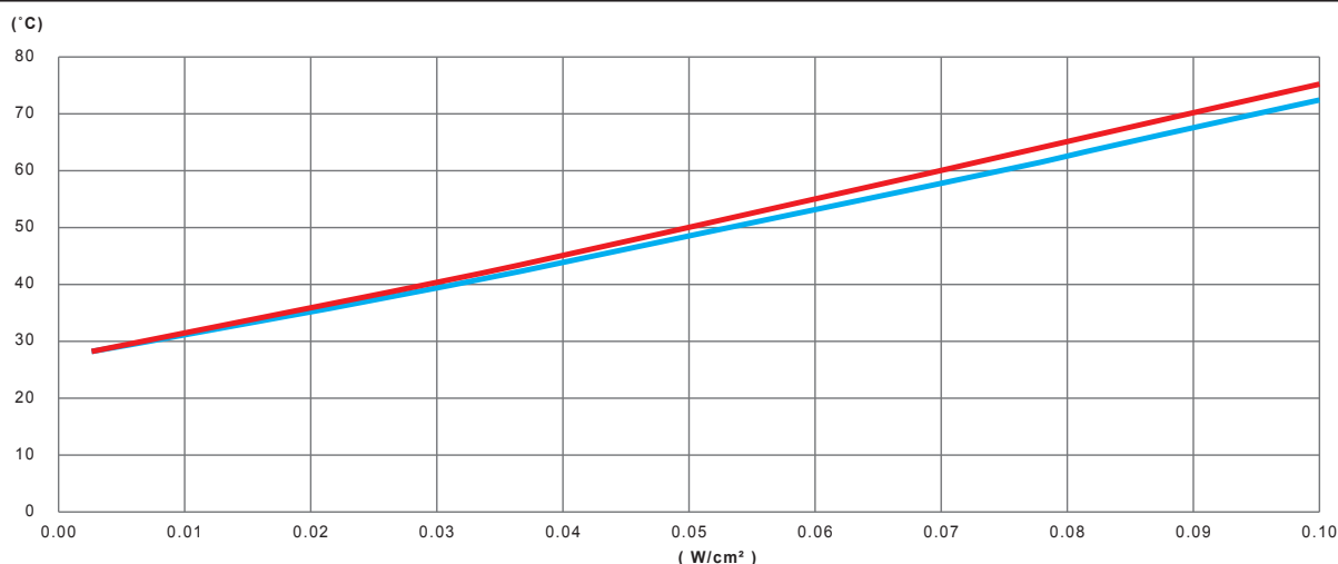
Variation, en fonction de la puissance en W/cm² du ruban chauffant en silicone, de la température de paroi d'un tube en PVC vide, isolé thermiquement par 20mm de mousse PVC-NBR
