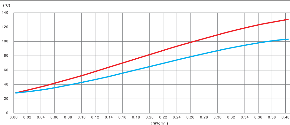
Variation, en fonction de la puissance en W/cm² du ruban chauffant en silicone, de la température de paroi d'un tube en PVC rempli d'eau non circulante, isolé thermiquement par 20mm de mousse PVC-NBR
